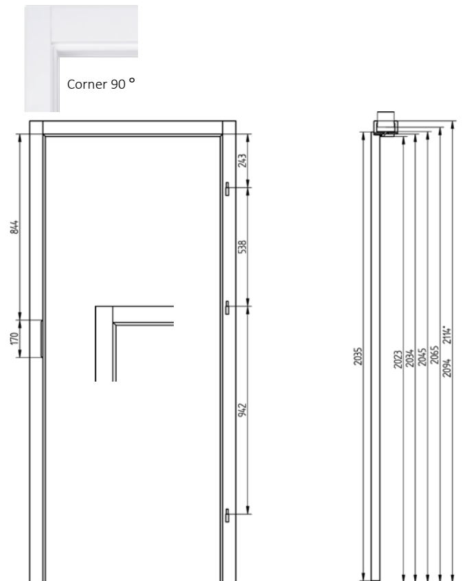
E2* - dimension for OW
