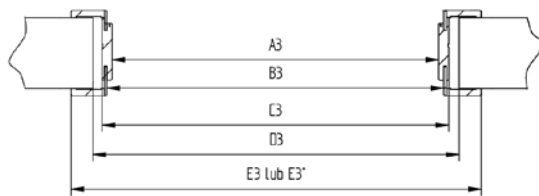
E3* - dimension for TW
