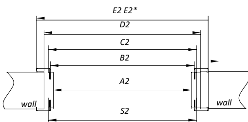
E2* - dimension for OW
