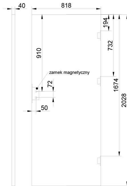
skrzydło bezprzylgowe
