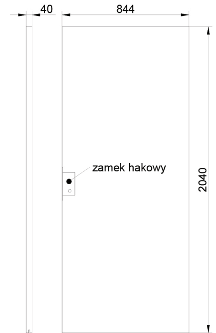
skrzydło przesuwne
