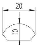
PRZEKRÓJ ĆWIERĆWAŁKA
