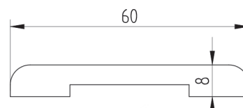
PRZEKRÓJ OPASKI MASKUJĄCEK
